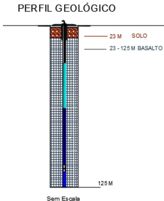
Figura 12: Perfil Geológico do Poço. Fonte: Autor (2022).
