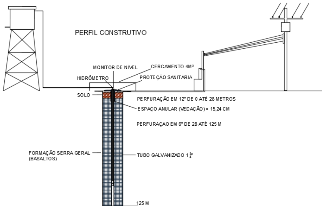
Figura 13: Perfil Construtivo do Poço. Fonte: Autor (2022).
