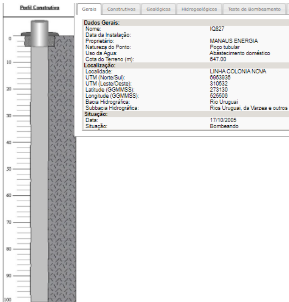
Figura 10: Perfil Geológico do Poço 1. Fonte: SIAGAS (2022).
