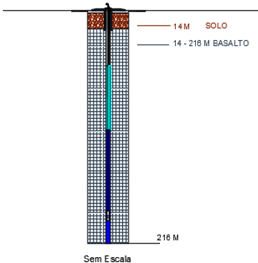
Figura 13: Perfil Geológico do Poço. Fonte: Autor (2022).
