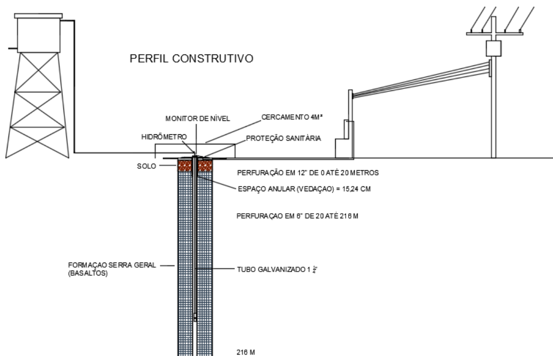
Figura 14: Perfil Construtivo do Poço. Fonte: Autor (2022).
