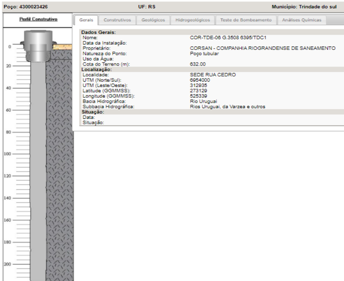
Figura 12: Perfil Geológico do Poço 3. Fonte: SIAGAS (2022).
