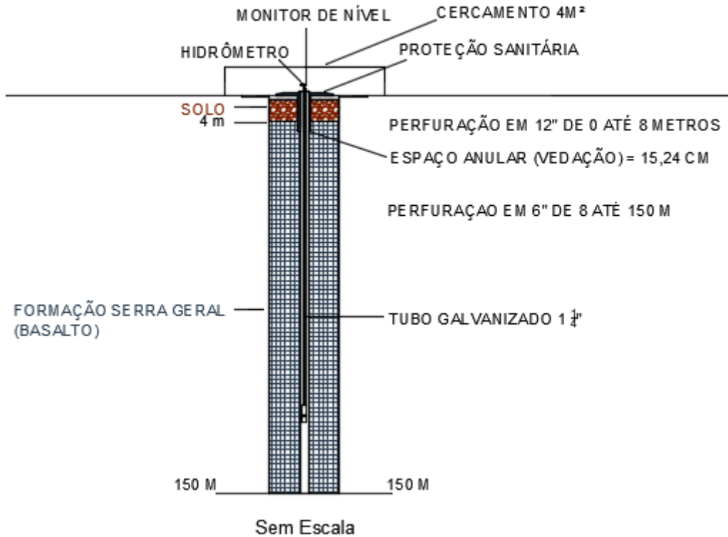
Figura 12: Perfil Geológico e Construtivo do Poço. Fonte: Autor (2024).
