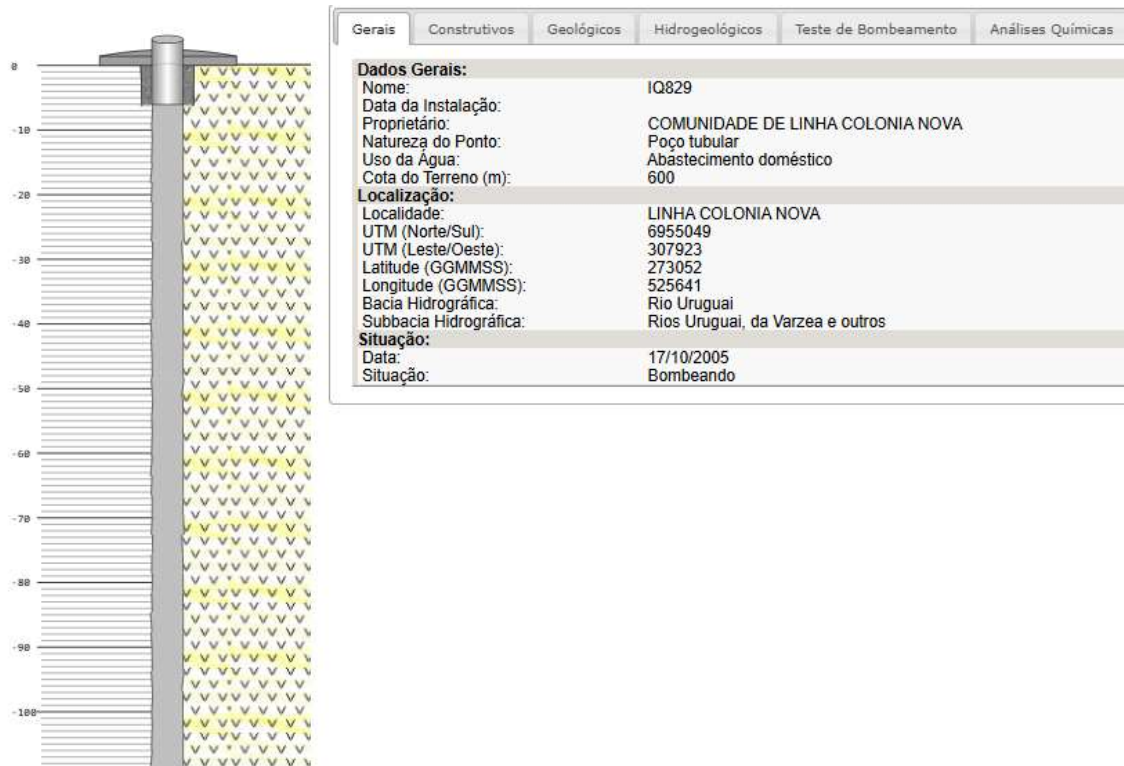
Figura 11: Perfil Geológico do Poço 2. Fonte: SIAGAS (2024).
