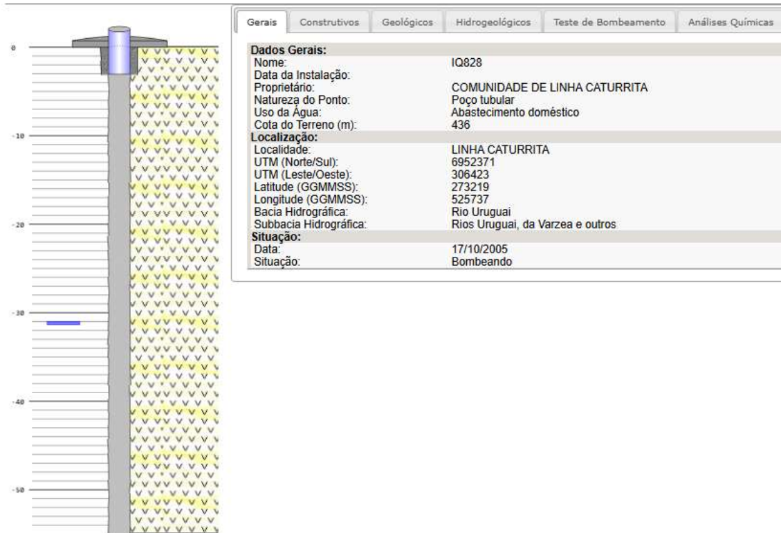
Figura 10: Perfil Geológico do Poço 1. Fonte: SIAGAS (2024).
